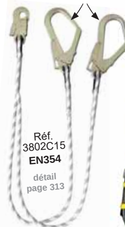
Mousquetons d'échafaudage Ouverture 55 mm
