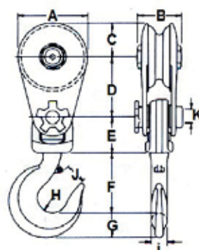
Crochet avec linguet de sécurité
