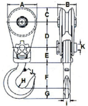
Crochet avec linguet de sécurité
