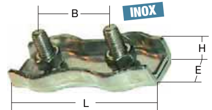
2 BOULONS Réf. 5287
