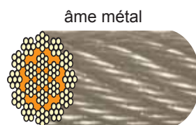
19 x 7 fils
