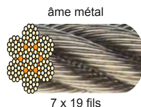
âme métal 7 x 19 fils
