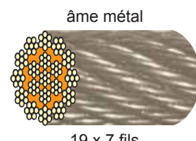
âme métal 19 x 7 fils
