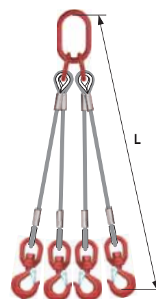
4 crochets à touret
