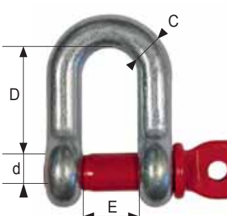
Réf 5220 : AXE À OEIL
