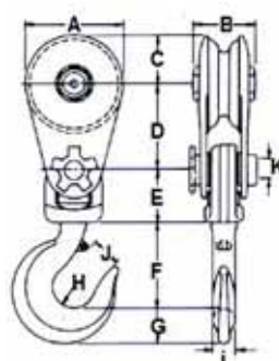
Réa bagué-bronze
