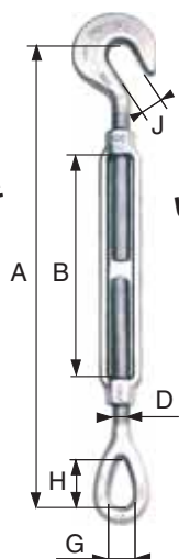
réf 5307/8 * 1 crochet 1 oeil
