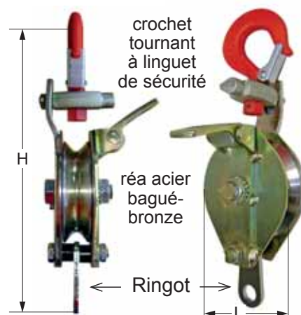
Modèle à 2 réas
