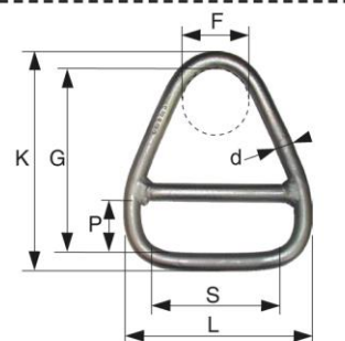
ANNEAU FEMELLE ref. 5072
