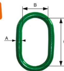
ANNEAU SIMPLE ref. 5058 Pour élingues-câble 1 et 2 brins
