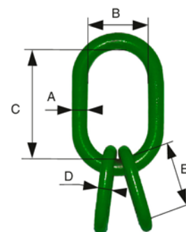
ANNEAU TRIPLE ref. 5059 Pour élingues-câble 3 et 4 brins
