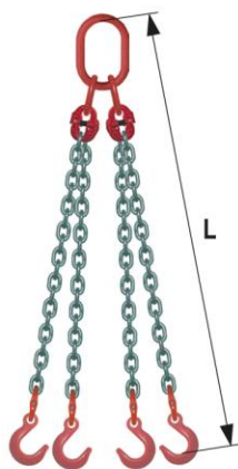
4 crochets de fonderie réf 4352
