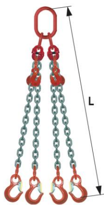
réglable à 4 crochets standard réf 4349 codes X à F
