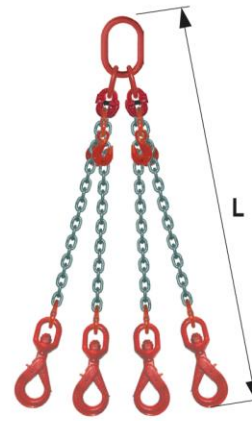
réglable à 4 crochets à touret verrouillage automatique réf 4357
