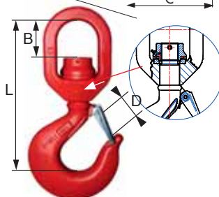
réf. 5131 MODÈLE avec ROULEMENTS Tournant sous charge
