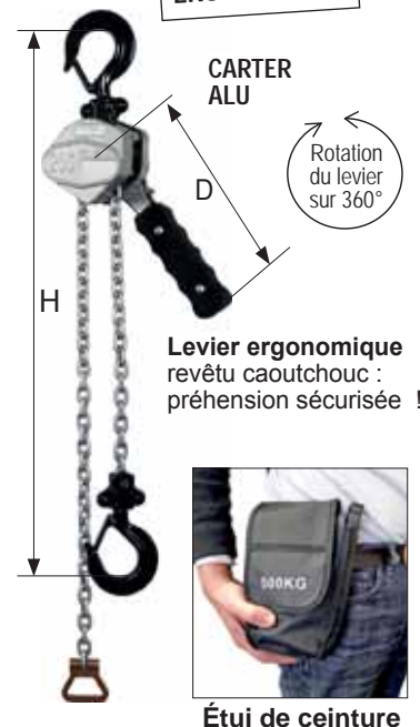
réf. 6047 Carter ALU codes A - B SANS limiteur de charge
