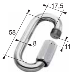
CMU : 700 kg Acier zingué Coef. sécu. 1/5 Poids : 0,078 kg
